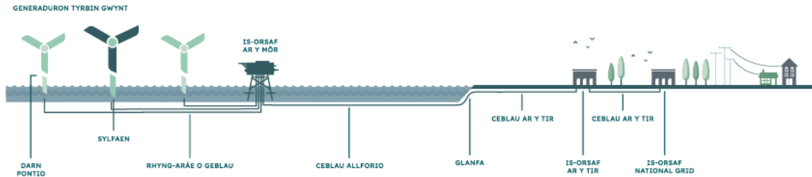
Ffigur 2: Cydrannau fferm wynt arferol ar y môr
